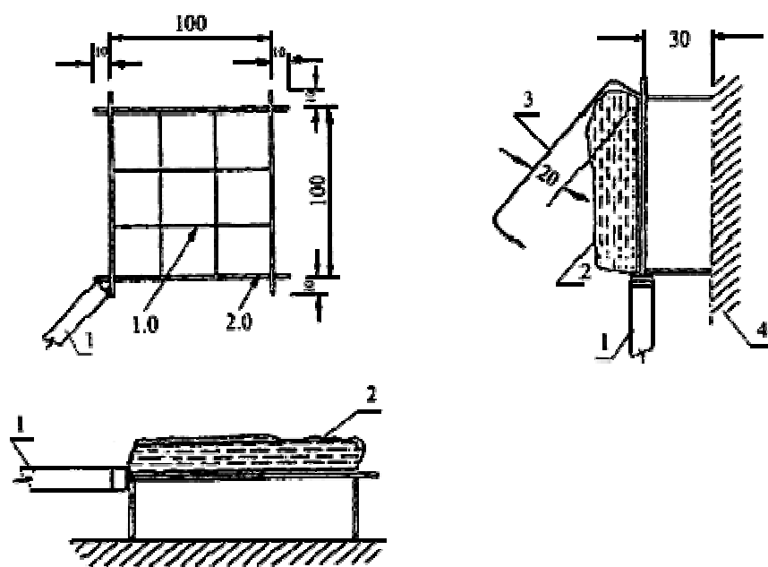
Рисунок Б.1 - Рамка для закрепления ватного тампона
