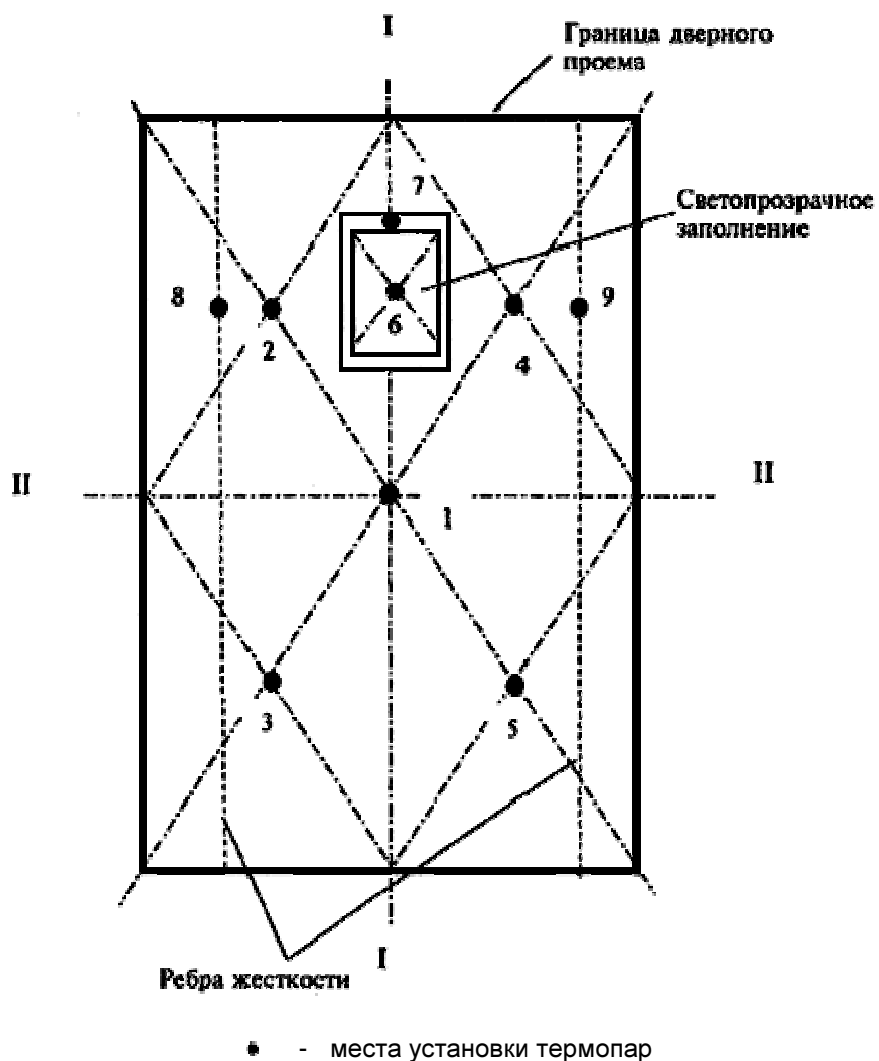
Рисунок А.1 - Схема установки термопар на необогреваемой поверхности створки одностворчатой
