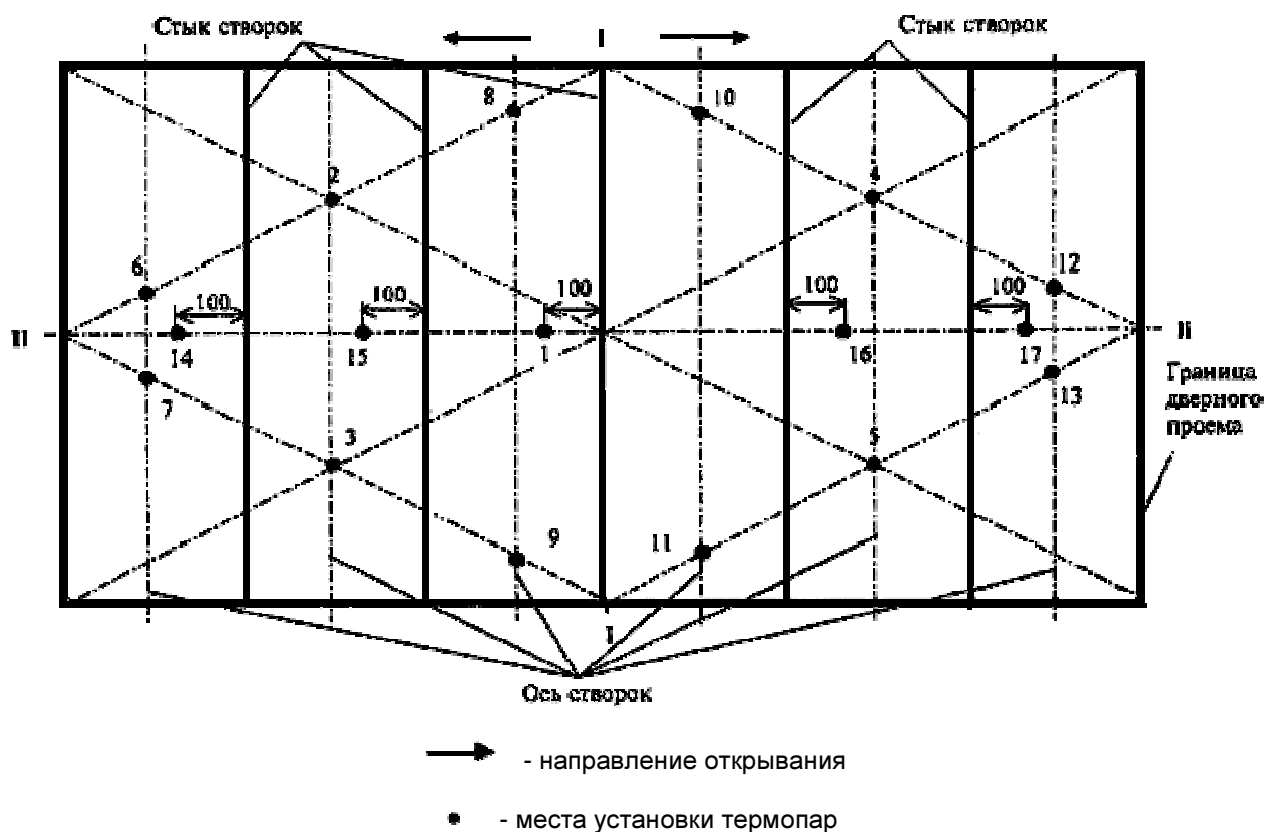
Рисунок А.5 - Схема установки термопар на необогреваемой поверхности шестистворчатой горизонтально-раздвижной двери центрального открывания
