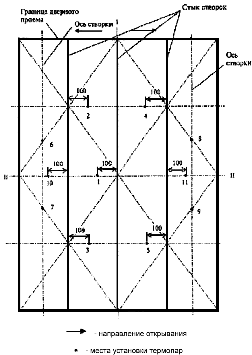
Рисунок А.4 - Схема установки термпар на необогреваемой поверхности четырехстворчатой горизонтально-раздвижной двери центрального открывания
