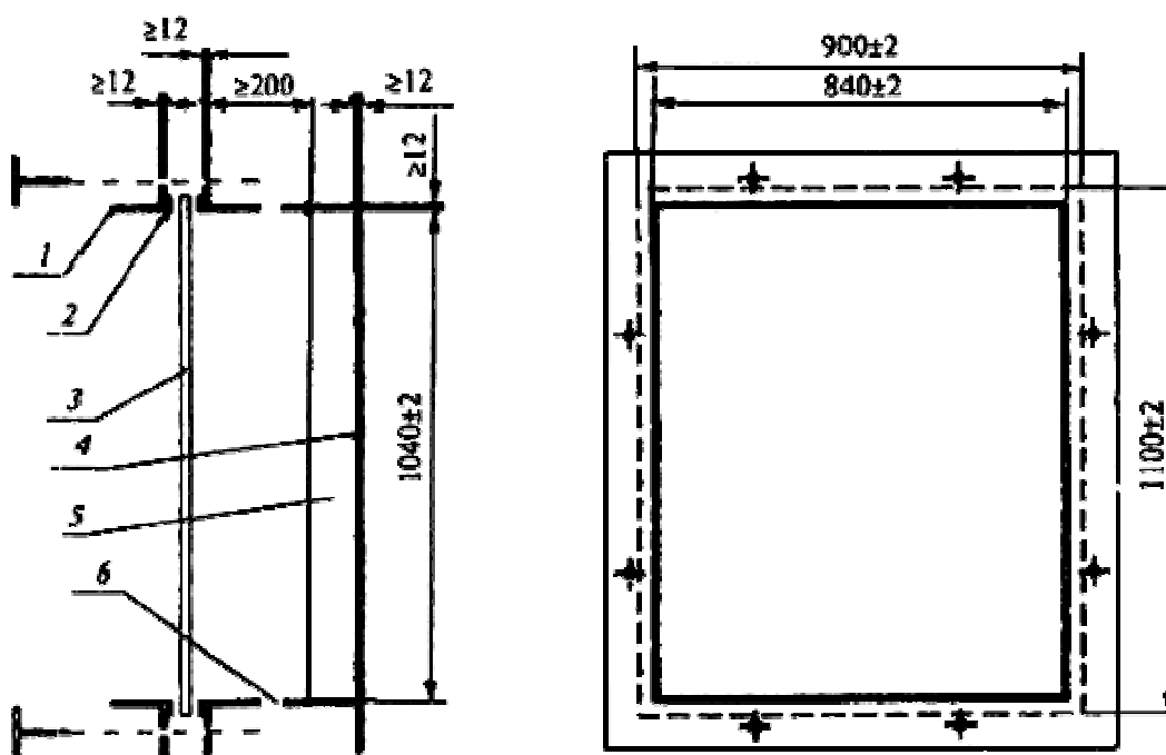
1 - стальная зажимающая рама; 2 - резиновая полоса; 3 - испытуемый образец; 4 - приемный ящик; 5 - мягкая прокладка; 6 - отверстие
