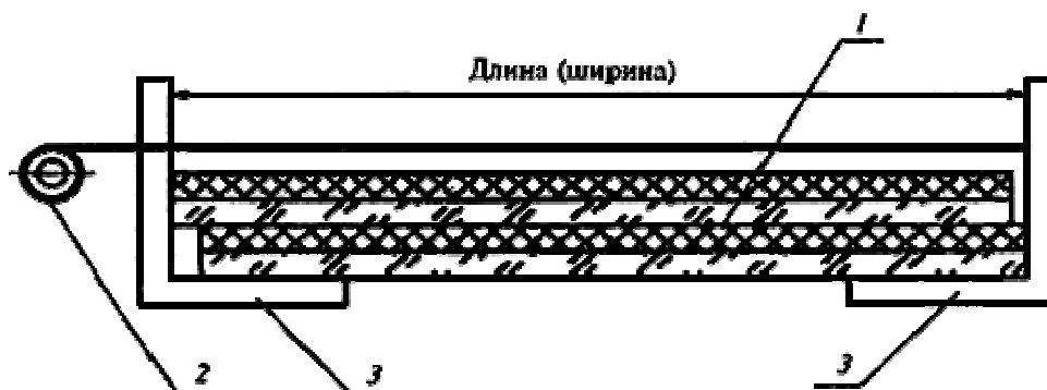
1 - многослойное стекло; 2 - рулетка; 3 - металлический угольник
