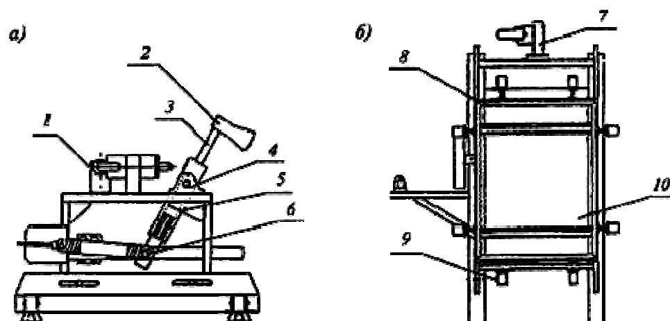
1 - высвобождающий механизм; 2 - головка топора; 3 - рукоятка; 4 - ось вращения; 5 - зажимное приспособление; 6 - натяжная пружина; 7- регулятор высоты; 8 - зажимная рама; 9 - пневматические зажимы; 10 - испытываемый образец
