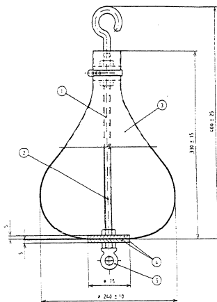
Рис. 2. Маятник для нежесткого удара
